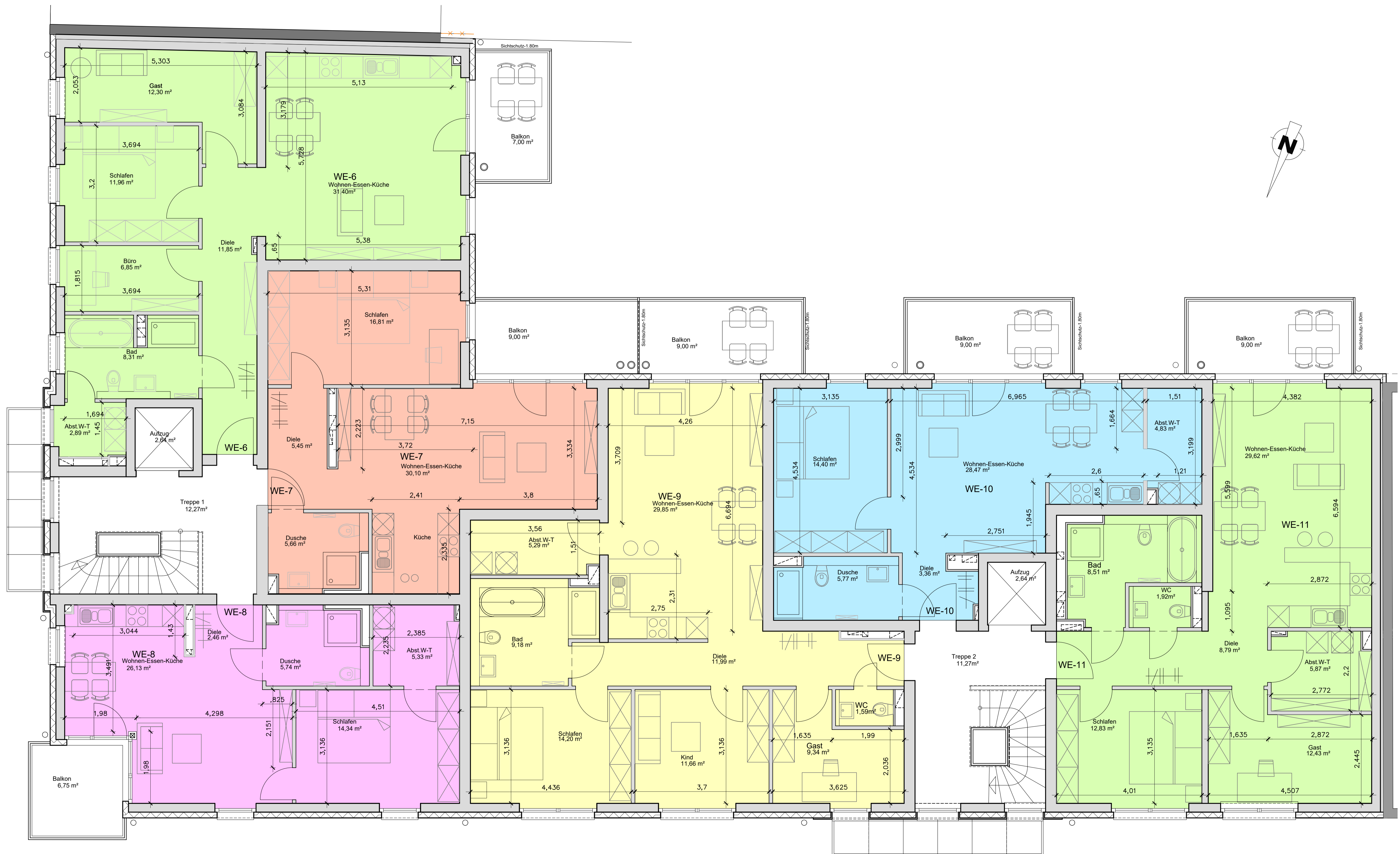
1. Obergeschoss
